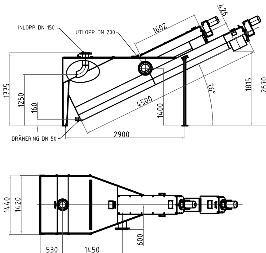
Standardritning DA 320.
